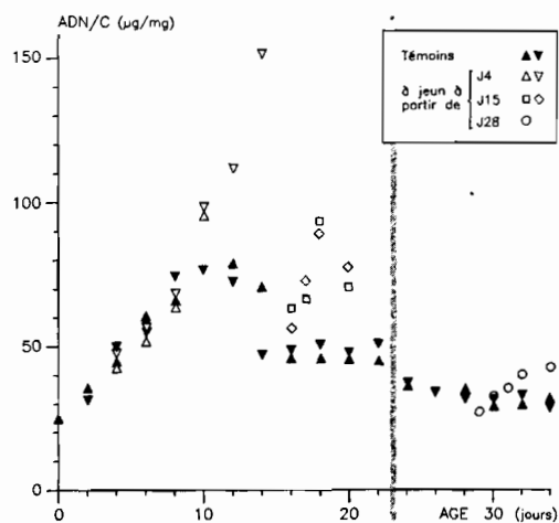
Figure 2. – Évolution de la teneur en ADN (en \mu\text{g.mg}^{-1} de carbone) de la larve de bar au cours de son ontogénèse (âge exprimé en nombre de jours après l'éclosion) et effet de la privation de nourriture à différents stades de développement. Un repère ombré à J23 indique le début de la flexion de la notochorde.
