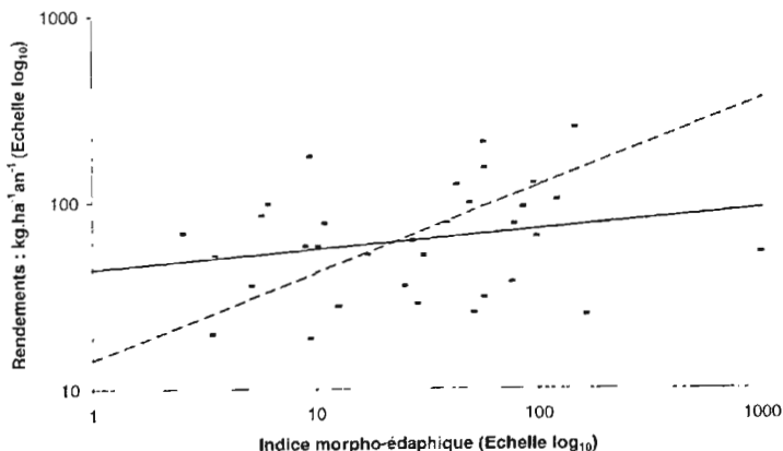
Figure 1. – Relations entre l'indice morpho-édaphique et les rendements de pêche (kg.ha -1 .an -1 ). ---- pour 33 lacs caractérisés par un effort de pêche supérieur à 1 pêcheur par km 2 (Henderson et Welcomme, 1974), ___ pour 65 lacs africains (Tableau 1).
