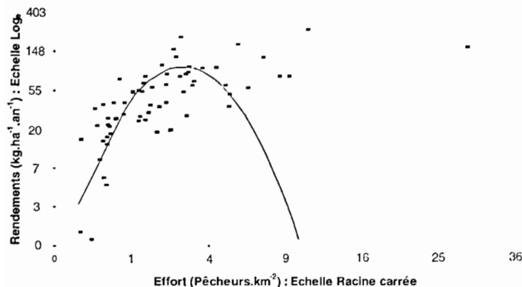
Figure 3. – Relation entre l'effort de pêche (pêcheurs.km 2 ) et les rendements de pêche (kg.ha -1 .an -1 ), pour 31 lacs africains (Bayley, 1988). ..... données provenant de 65 lacs africains (Tableau 1).
