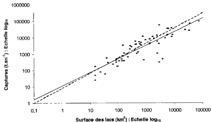
Figure 2. – Relations entre la surface (km 2 ) et les captures annuelles (t.an -1 ). --- pour 71 lacs (Crul, 1992), ___ pour 65 lacs africains (Tableau 1).
