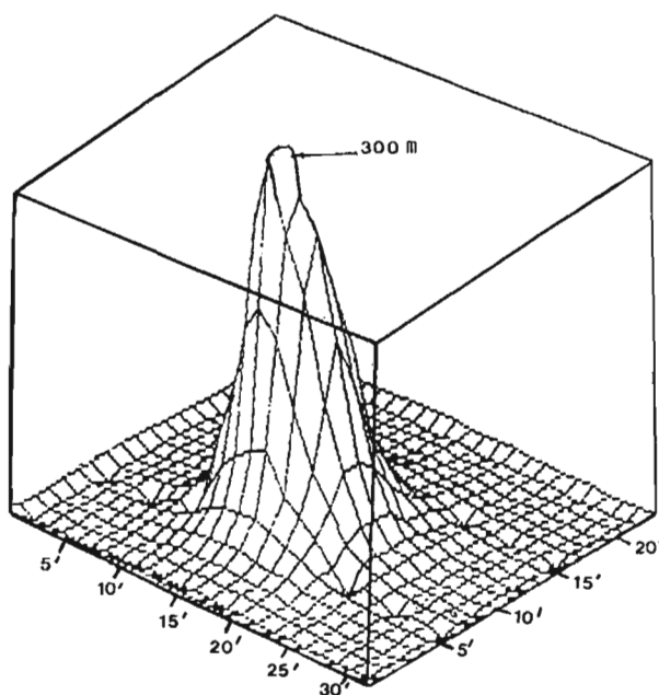
Figure 1. — Représentation schématique tridimensionnelle du mont sous-marin numéro 1 (situé au N.E. de l'île de Sal).
