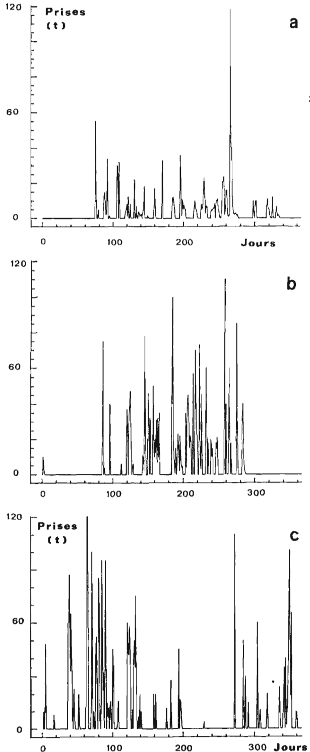
Figure 5. — Prises totales journalières (toutes flottilles, toutes espèces) observées sur le mont sous-marin 11 en 1981, (a) sur le mont sous-marin 11 en 1984, (b) et sur le mont sous-marin 20 en 1984 (c).
