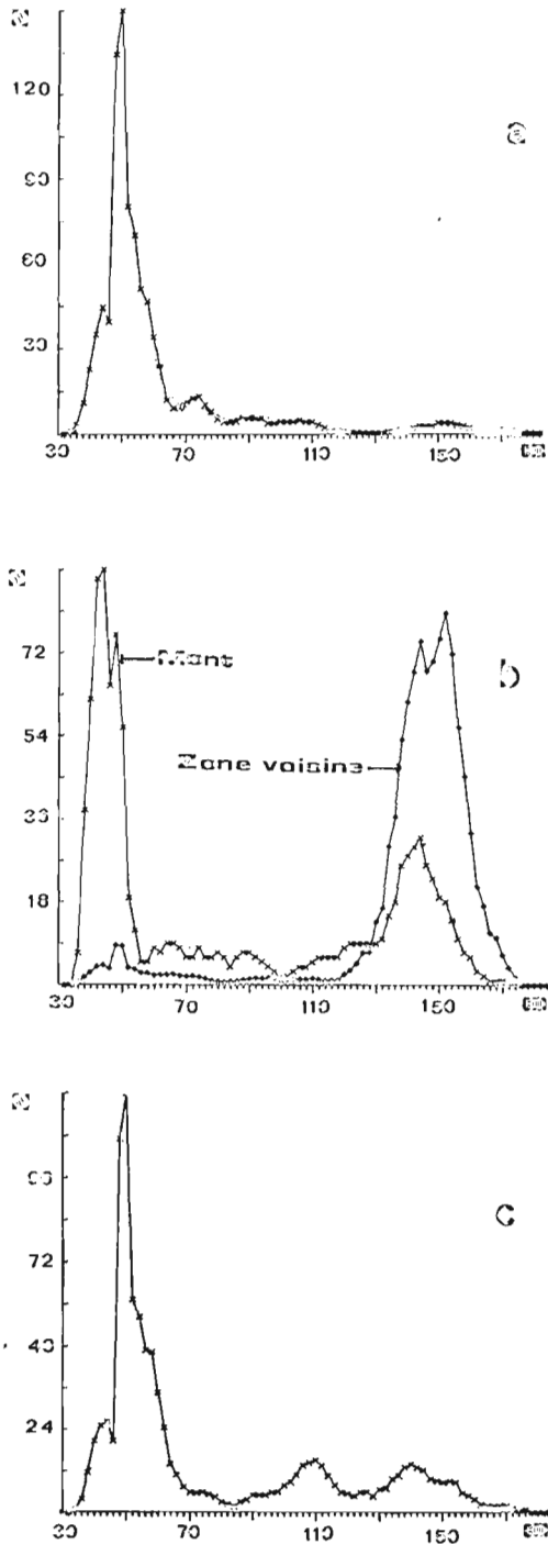
Figure 6. — Fréquences de tailles des captures d'albacore durant la période 1980 à 1987, (a) pour le mont sous-marin 11 (senneurs + -canneurs), (b) pour le mont sous-marin 20 (senneurs) et dans les deux zones de 5° adjacentes, (c) pour les albacores pêchés sous épaves flottantes (1980 à 1982).
