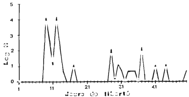
Figure 8. — Évolution du nombre de recaptures journalières durant les 50 jours après les marquages (échelle logarithmique), toutes espèces, sur le mont sous-marin 11 (même position qu'au marquage).
