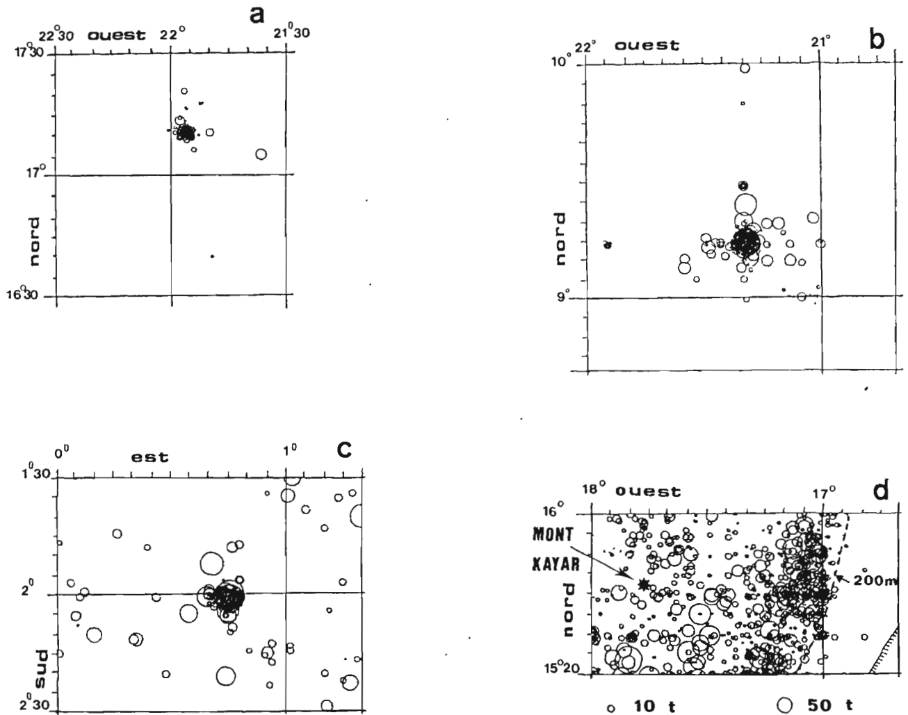
Figure 3. Prises observées de 1980 à 1987, dans la zone du mont sous-marin 1 (a), dans la zone du mont sous-marin 11 (b), dans la zone du mont sous-marin 20 (c), dans la zone du mont sous-marin 4 (d), (localisation des prises connue au mille près).
