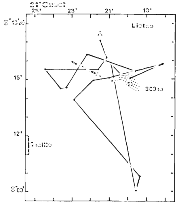
Figure 7. — Déplacements horizontaux du listao marqué durant 44 heures avec un microémetteur sur le mont sous-marin 11 (D) en octobre 1981, --→ courant (Lévénez, 1982).
