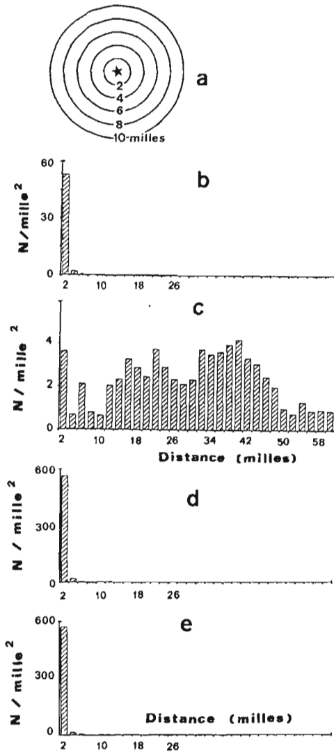
Figure 4. — Prises totales observées de 1980 à 1987 par unité de surface de 1 mille carré pour 30 cercles concentriques (a) situés autour des monts sous-marins 1, 4, 11 et 20, (b) à (e) pour des distances accrues selon un pas de 2 milles.
