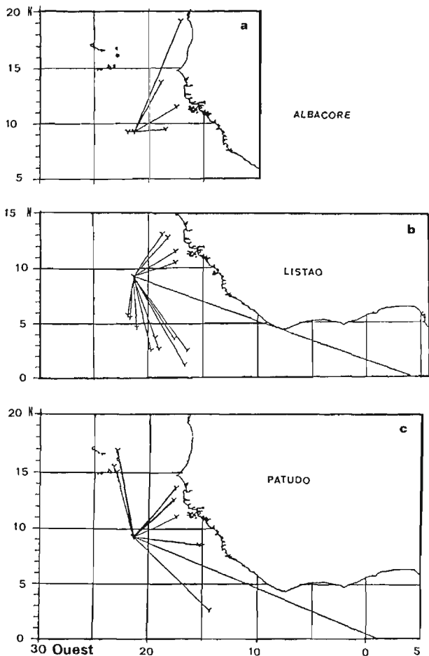
Figure 9. — Migrations apparentes des thons ayant quitté le mont sous-marin 11 où ils avaient été marqués (a) albacore, (b) listao, (c) patudo.
