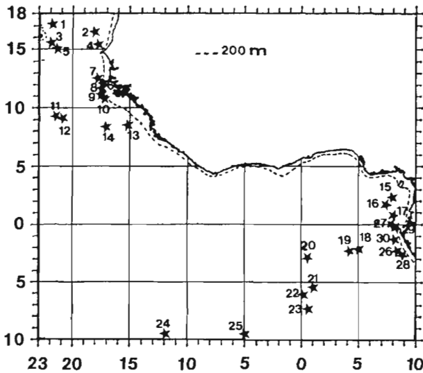
Figure 2. — Localisation et numérotation des 30 monts sous-marins analysés dans la présente étude.
